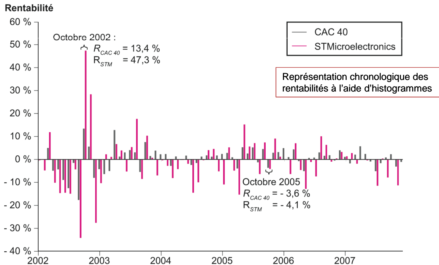
Fig12.6 (B&DM-p.404) : Rentabilités mensuelles de STMicroelectronics et du CAC40 sur 2002-2007
