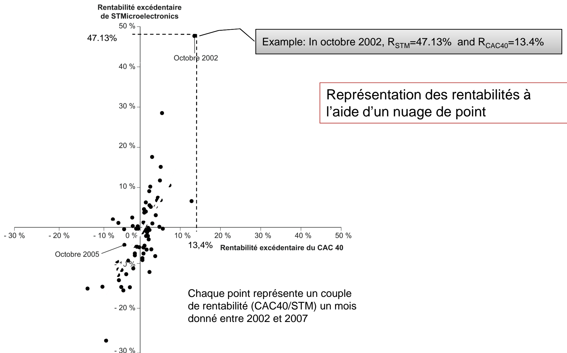
Fig12.6 (B&DM-p.404) : Graphique en nuage de points des rentabilités mensuelles de STMicroelectronics et du CAC40 sur 2002-2007
