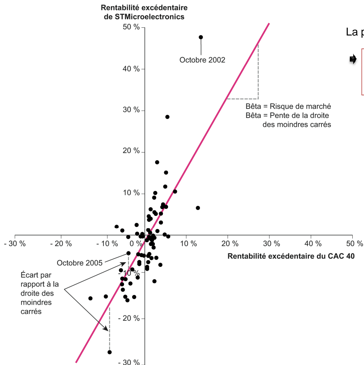
Fig12.6 (B&DM-p.404) : Graphique en nuage de points des rentabilités mensuelles de STMicroelectronics et du CAC40 sur 2002-2007
