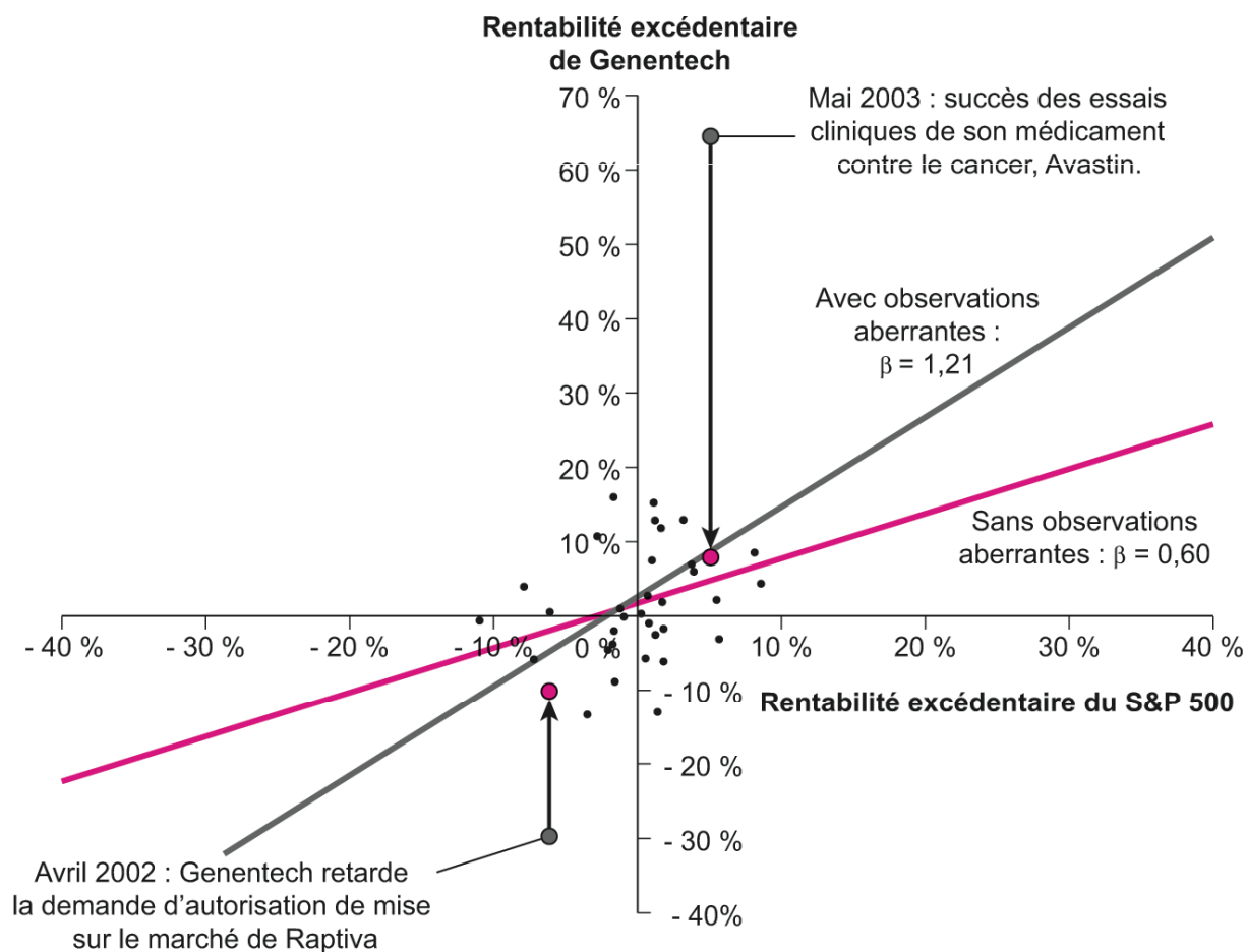
Fig12.10 (B&DM-p.414) : Estimation du bêta de DNA selon que les observations aberrantes sont, ou non, prises en compte
